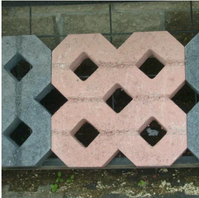
Adopasto Rombo 1 piezas por tarima
